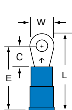
MNG14-4R/S Stud Size 4 Wire Range 16-14
