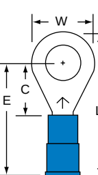
MNG14-14R/S Stud Size 1/4 Wire Range 16-14
