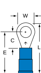
MNG14-10R Stud Size 10 Wire Range 16-14
