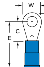
MNG14-8R/L Stud Size 8 Wire Range 16-14
