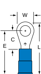
MNG14-10R/L Stud Size 10 Wire Range 16-14
