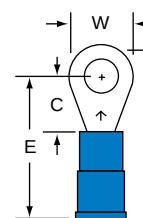
MNG14-8R Stud Size 8 Wire Range 16-14
