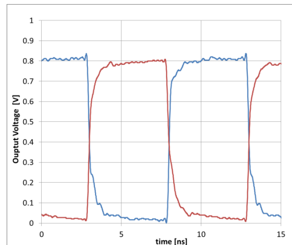
Figure 26. 100MHz HCSL
