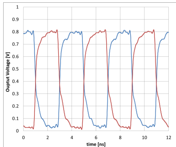
Figure 27. 250MHz HCSL
