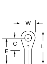
MU18-4R/S Stud Size 4 Wire Range 22-18
