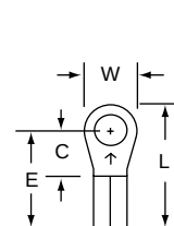
MU14-6R/S Stud Size 6 Wire Range 16-14
