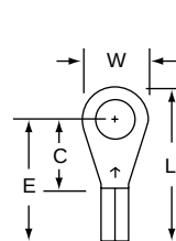
MU18-10R/L Stud Size 10 Wire Range 22-18
