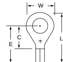
MU14-14R/S Stud Size 1/4 Wire Range 16-14
