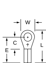
MU18-6R/S Stud Size 6 Wire Range 22-18
