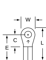
MU14-4R/S Stud Size 4 Wire Range 16-14
