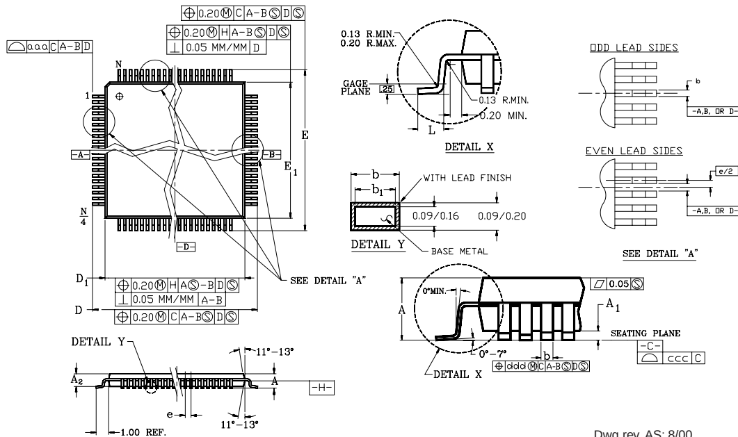
LQFP 064
